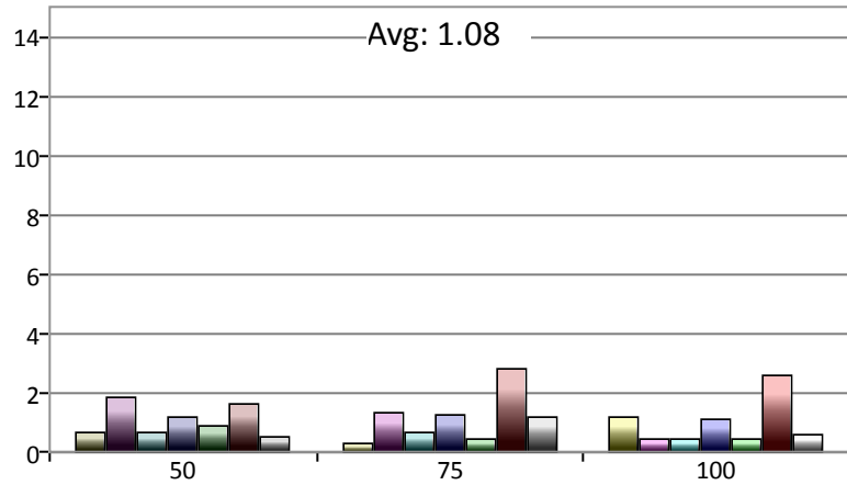
DeltaE 2000
